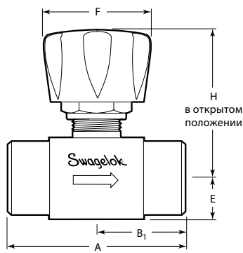
Прямая конфигурация
