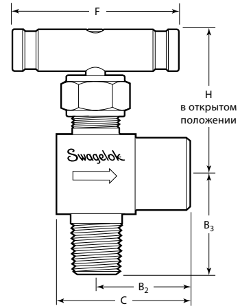
Угловая конфигурация
